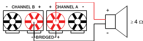
Abbildung 2.17: Lautsprecheranschluss in Betriebsart BRIDGED an Anschlussklemmen
